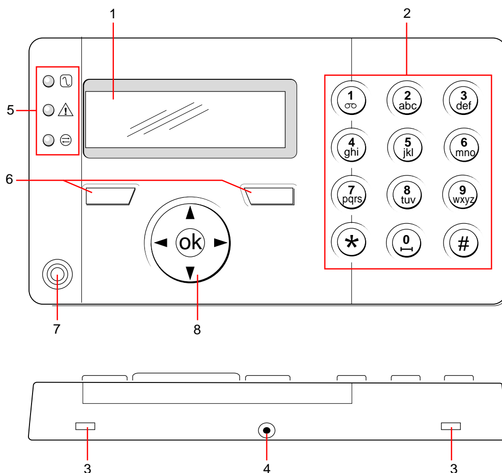
LCD-bediendeel
